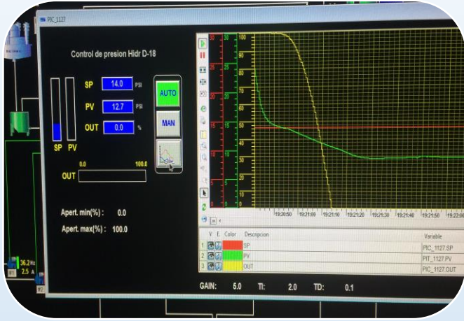
INTEGRACIÓN DE BOMBAS 250HP A SISTEMA SCADA EN UNIDAD MINERA CATALINA HUANCA
